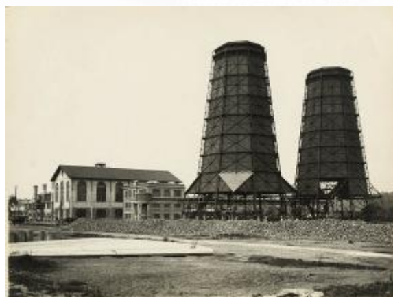
Référence : D23-41 Construction de l'usine de cyanamide de Carmaux. 23 mai 1918. Photographe inconnu/© ECPAD - Collection Mettra
